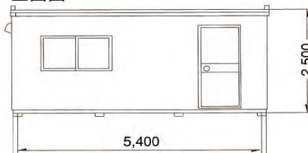
正面図
